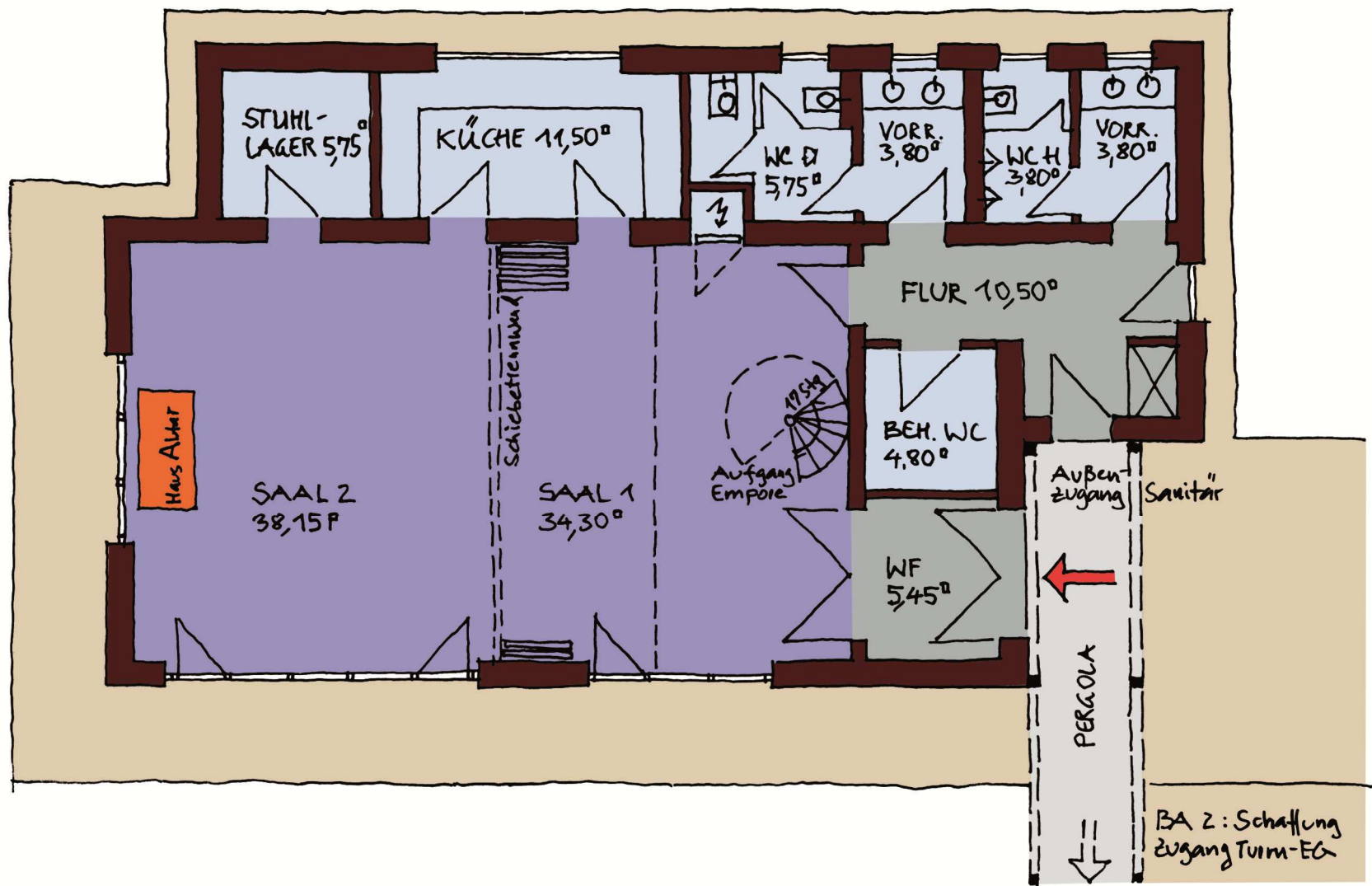
Grundriss ERDGESCHOSS
